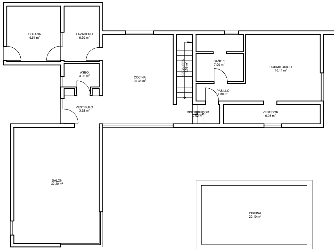
PLANTA BAJA
