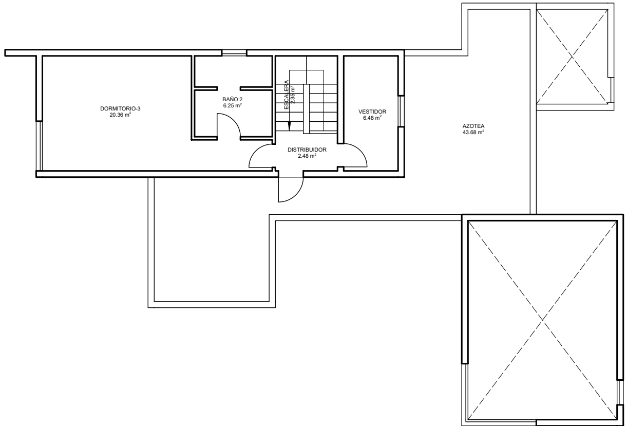
PLANTA ALTA
