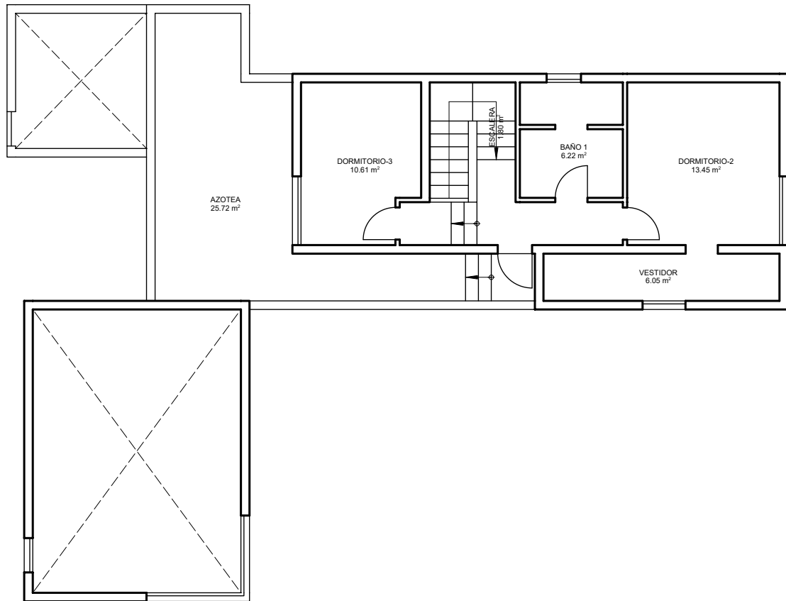
PLANTA ALTA
